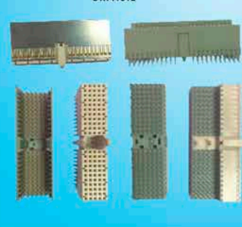
DIN41612
