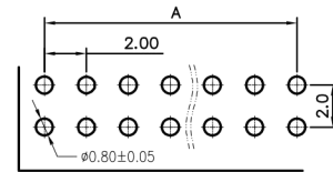
P.C.B. LAYOUT
